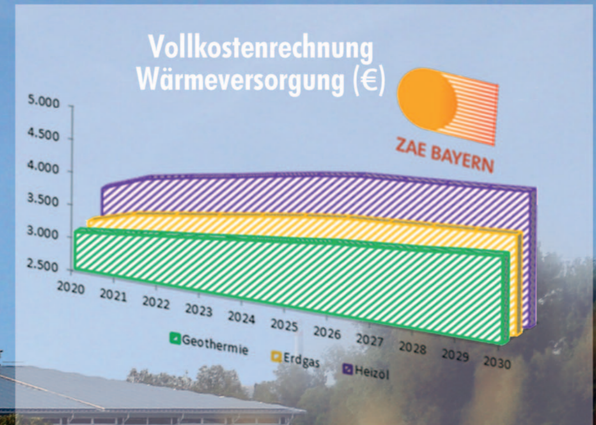
Eigene Darstellung der Vollkostenrechnung Geothermie im Vergleich zu Erdgas und Heizöl für einen Anschluss mit 20 kW (Annahme: CO 2 -Bepreisung von max. 60€ / t)
