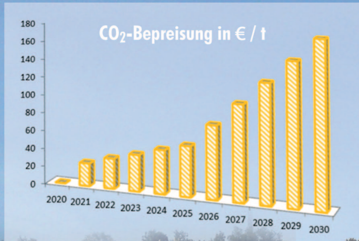
Eigene Darstellung der prognostizierten CO 2 -Bepreisung gemäß DIW-Studie
